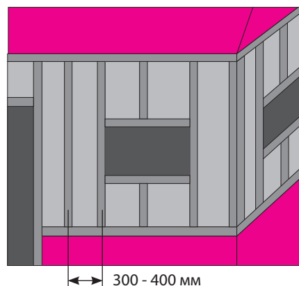
рис. 2 Вертикальная обрешетка
