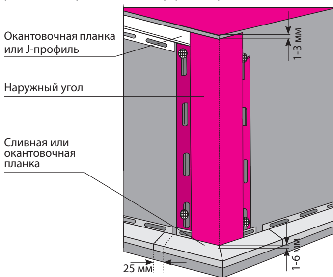
рис. 27 Схема установки аксессуаров и вертикального сайдинга
