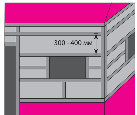
рис. 26 Горизонтальная обрешетка
